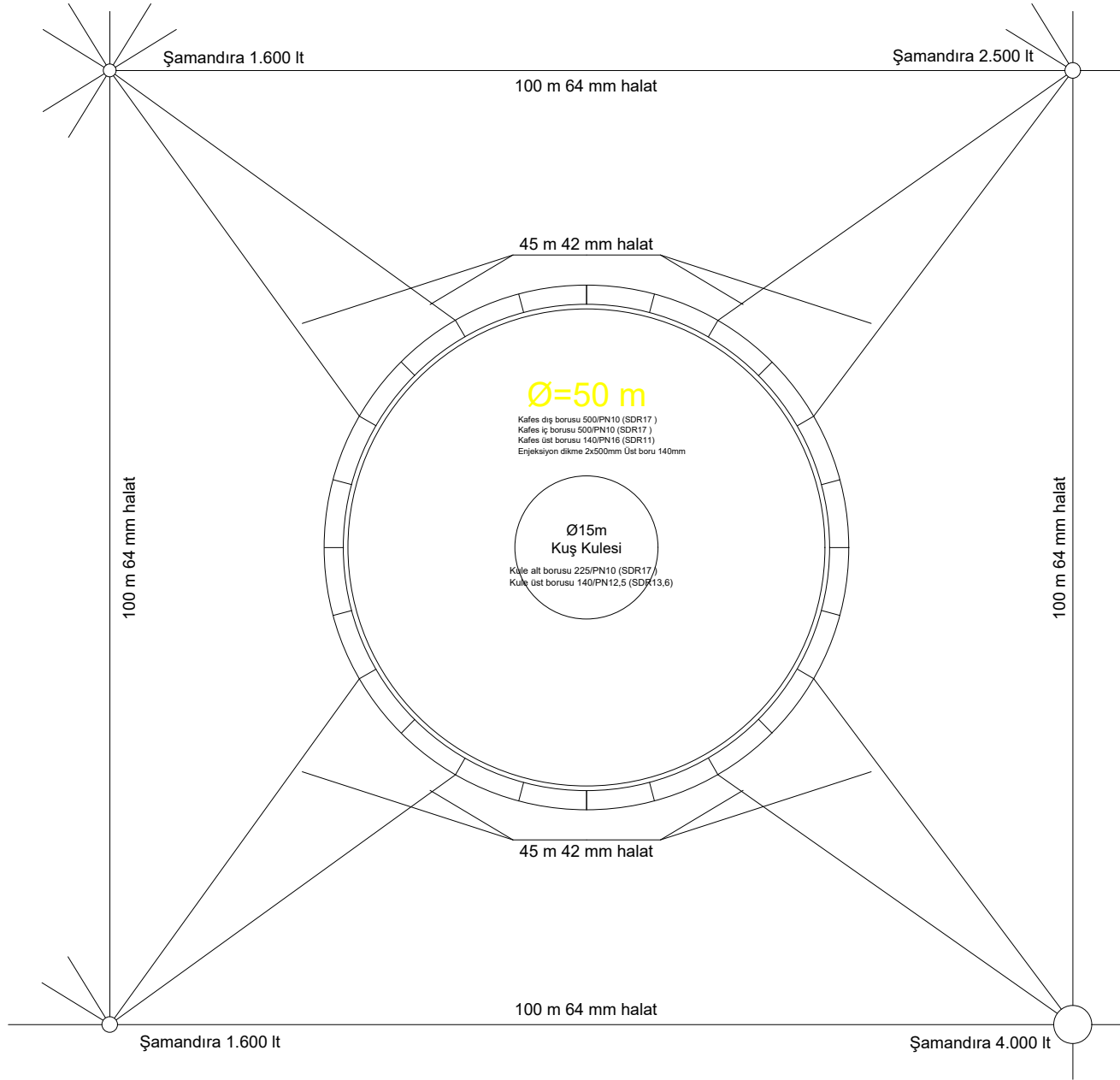
50,00 m. Çaplı, Dairesel, HDPE, Yüzer Ağ Kafes Üst Kesiti
